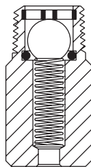
Fig. 2-4. Pop Drain
