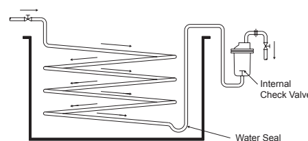
Fig. 1-7. Trap draining syphon.
